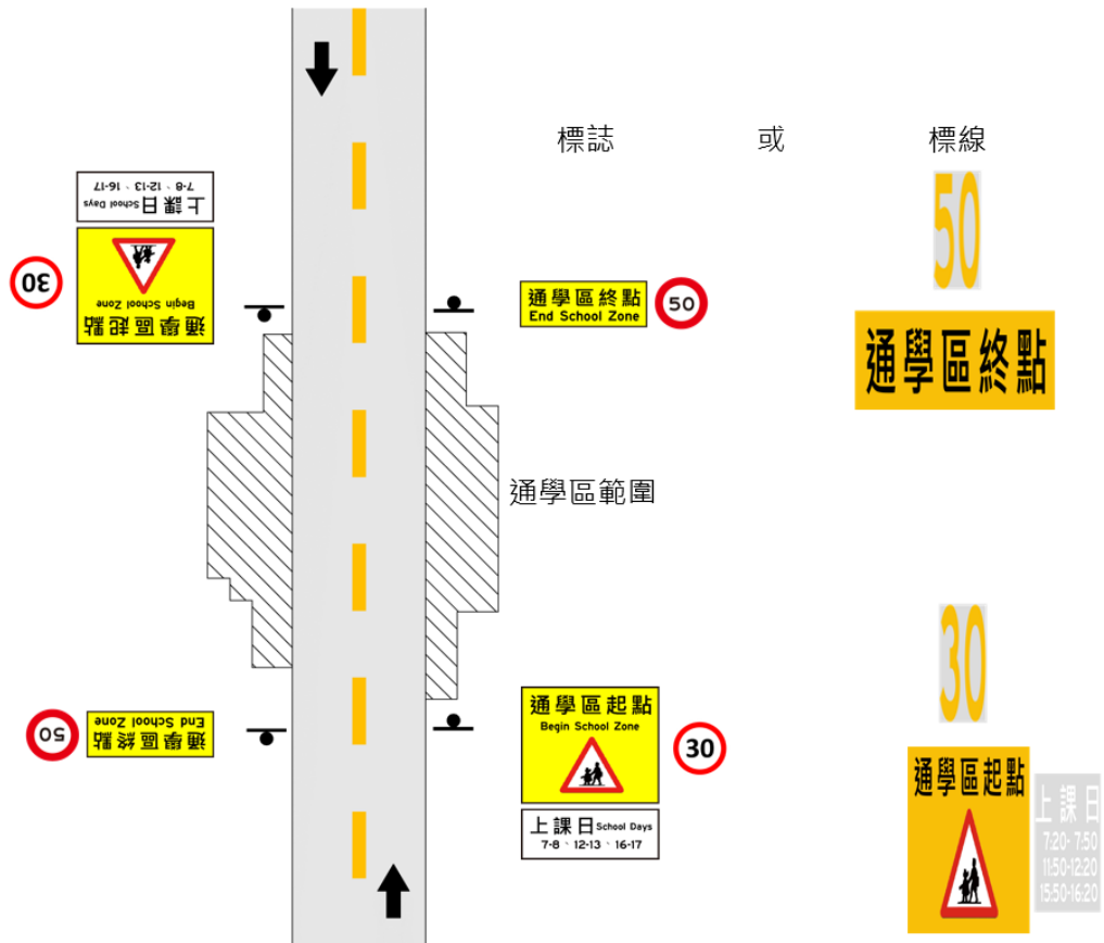
附錄圖 5 進出通學區範圍之通學區標誌（線）設置示意圖
