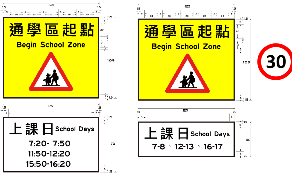
附錄圖 1 進入通學區標誌
