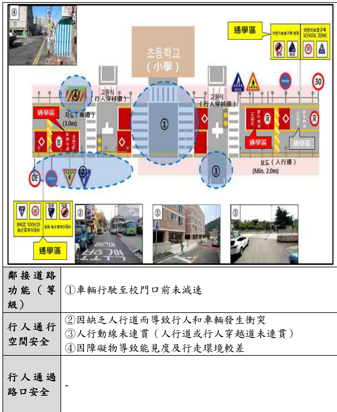
圖 2-2-42 地方道路 Type-B 之問題
