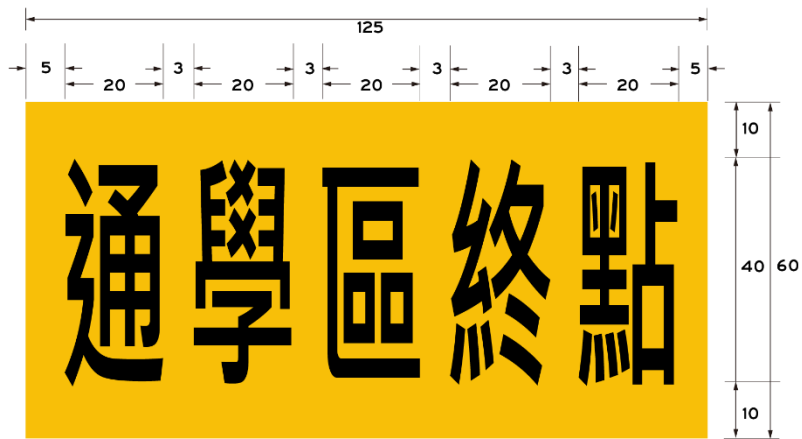
附錄圖 4 離開通學區標線
