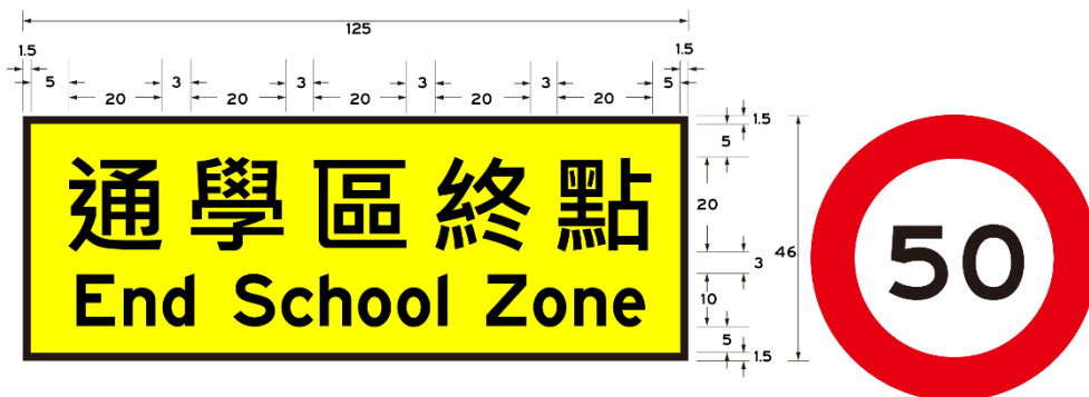
附錄圖 2 離開通學區標誌
